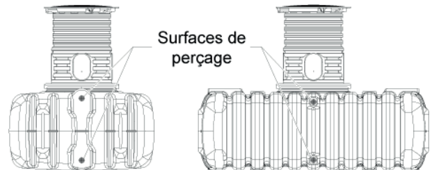
Fig. 25 : Surface de perçage pour relier plusieurs cuves – FLAT.
