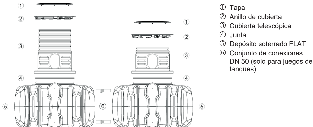
Fig.11: Componentes – FLAT
