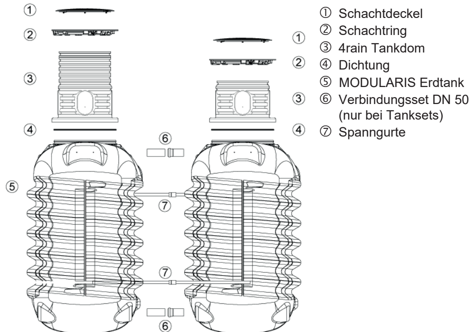
Abb. 18: Komponenten – MODULARIS
