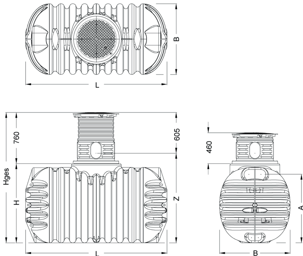
Abb. 9: Abmessungen – COMPACT
