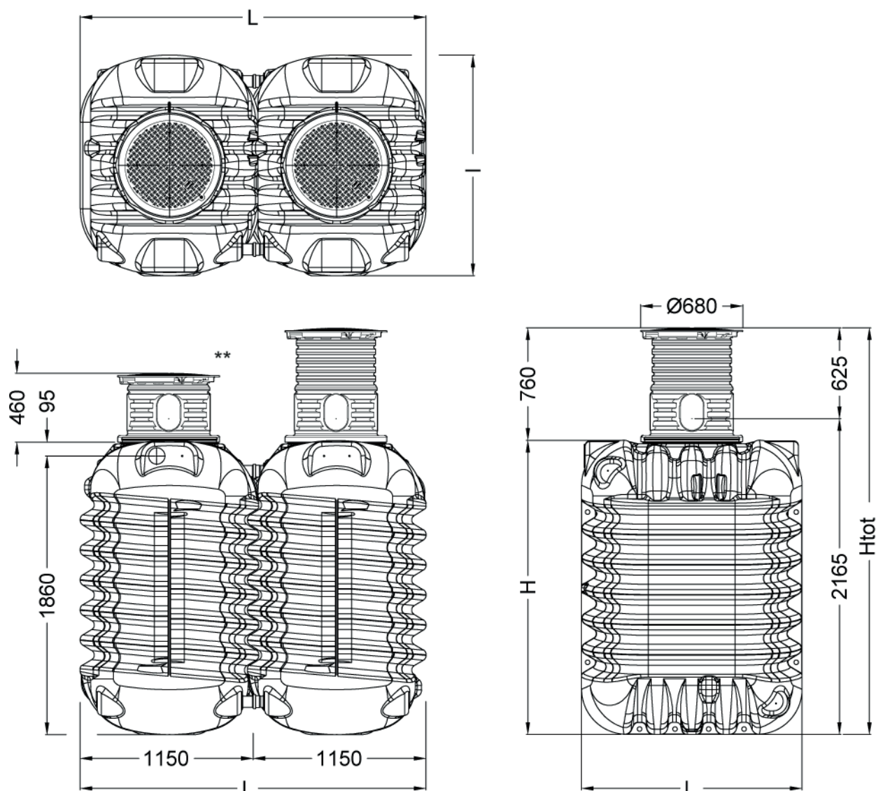
Fig. 8 : Dimensions – MODULARIS
