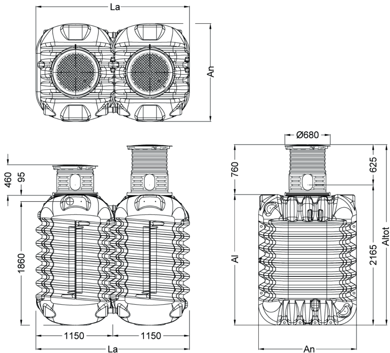
Fig.8: Dimensiones – MODULARIS
