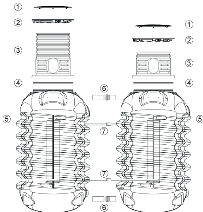
Fig. 18 : Composants – MODULARIS
