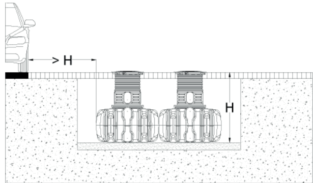
Fig. 24 : Distance par rapport aux surfaces de passage véhicules – Exemple FLAT
