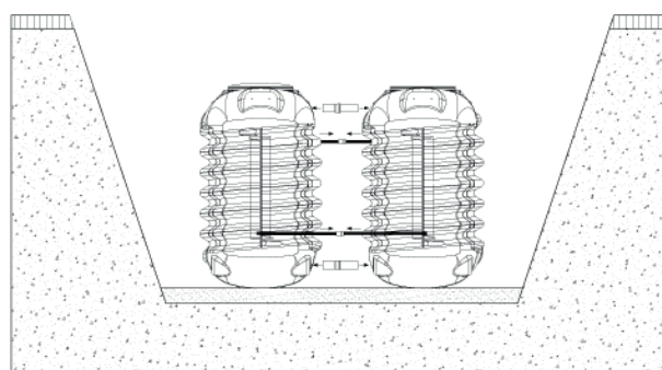
Fig. 27 : Jumelage de plusieurs cuves – MODULARIS
