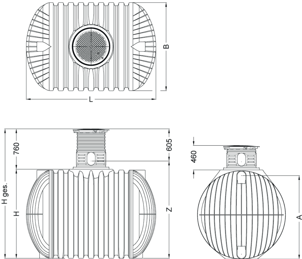
Abb. 10: Abmessungen – PROFI
