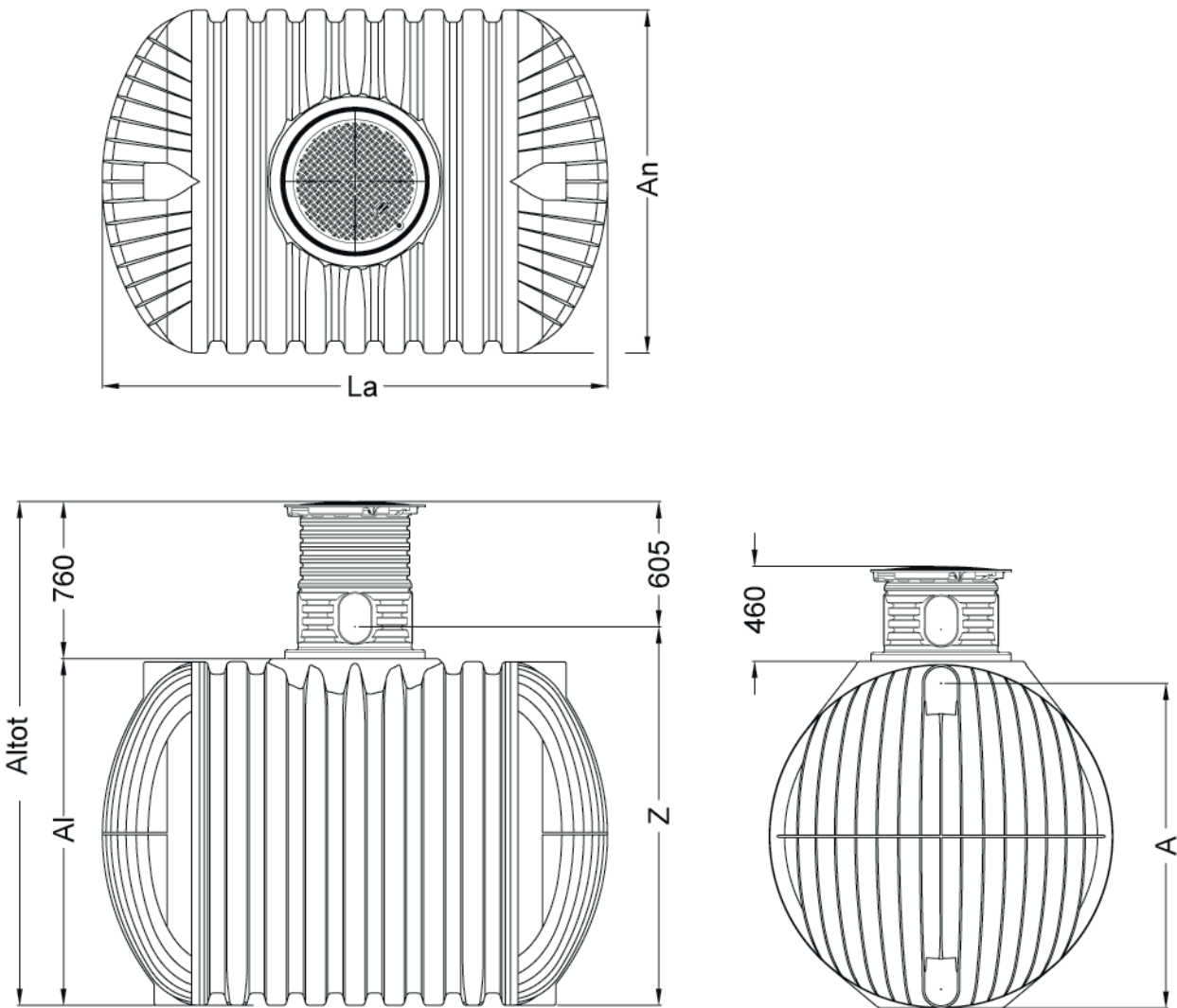
Fig. 10: Dimensiones – PROFÍ
