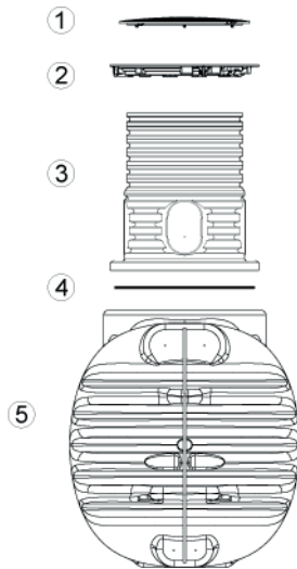
Abb. 19: Komponenten – COMPACT
