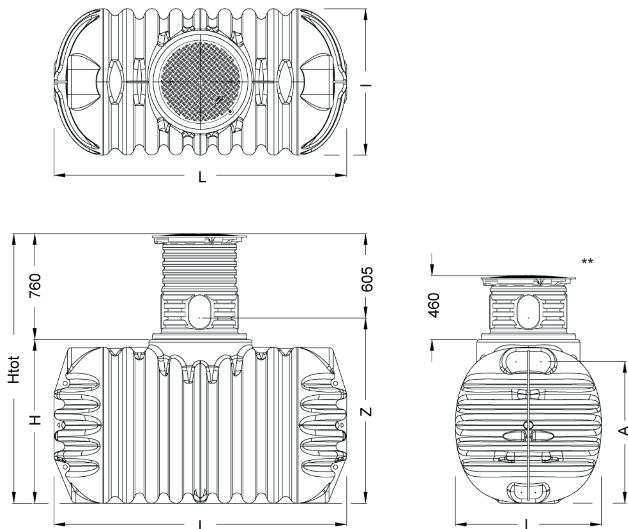
Fig. 9 : Dimensions – COMPACT
