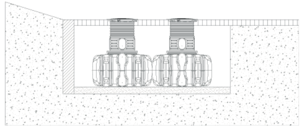
Fig. 22 : Installation sur terrain en pente – Exemple FLAT
