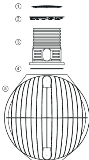
Abb. 20: Komponenten – PROFI
