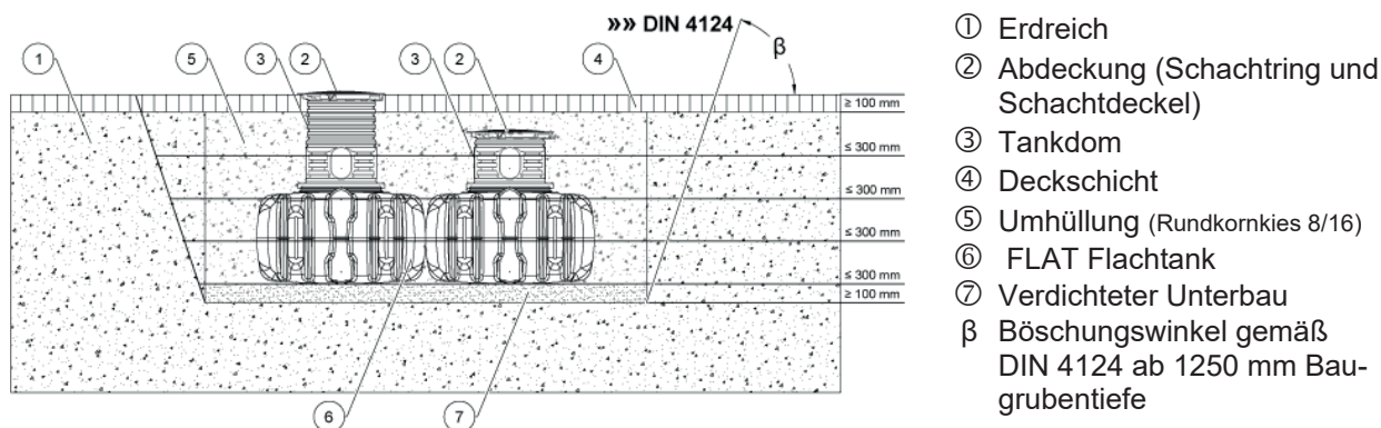
Abb. 21: Einbauschema – Beispiel FLAT
