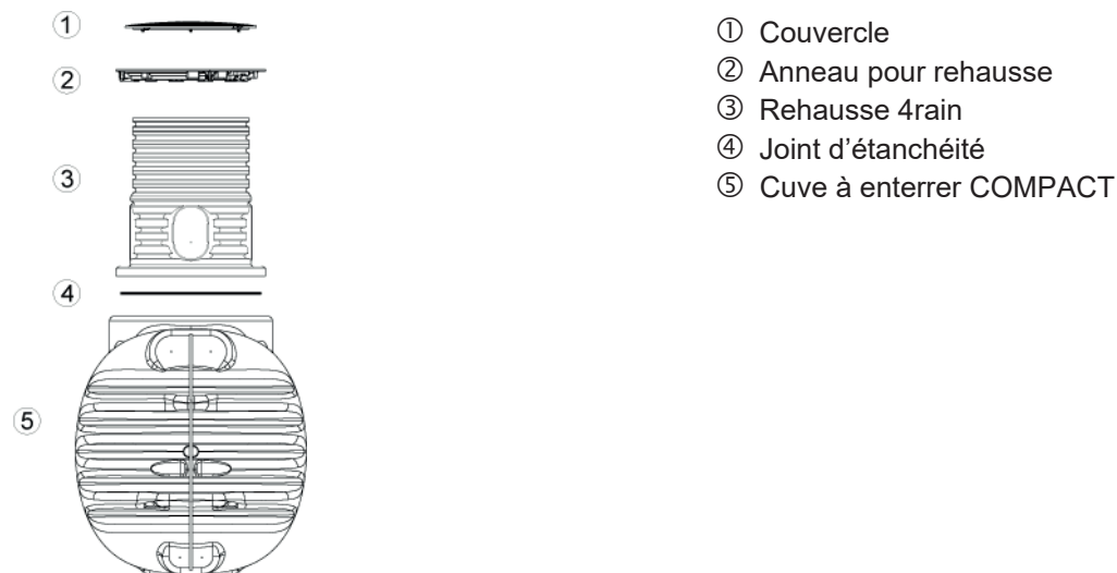
Fig. 19 : Composants – COMPACT
