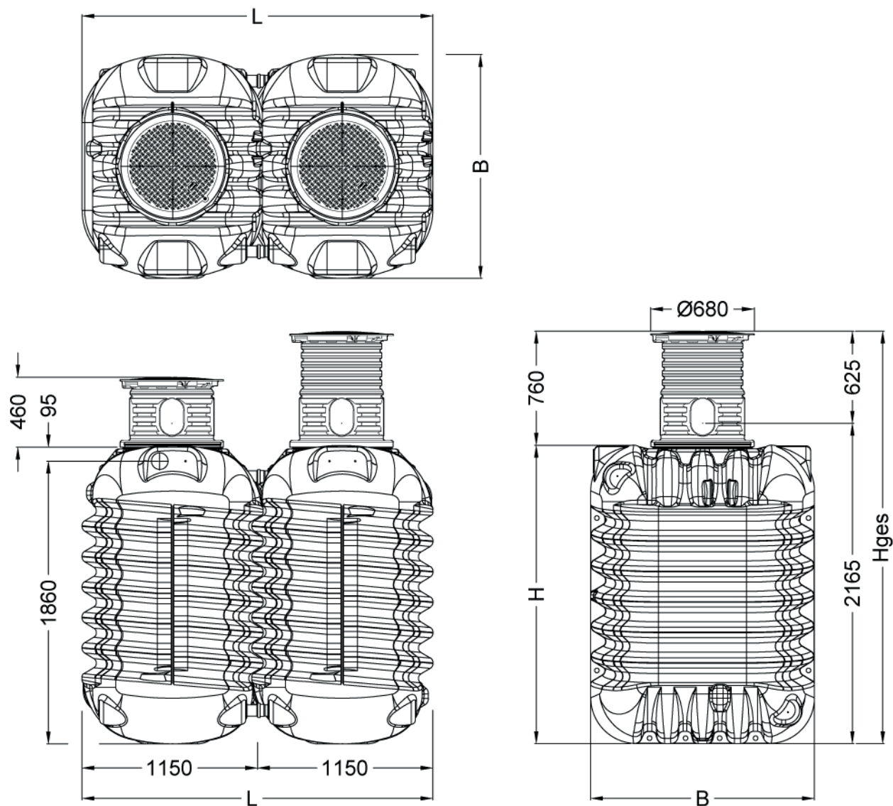
Abb. 8: Abmessungen – MODULARIS
