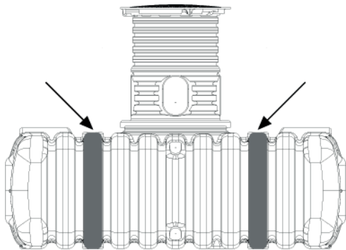
Fig. 12 : Vue en coupe des tubes de renfort– FLAT S/M
