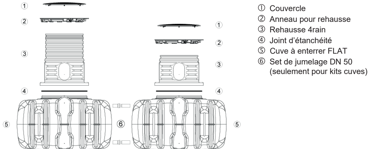
Fig. 11 : Composants – FLAT
