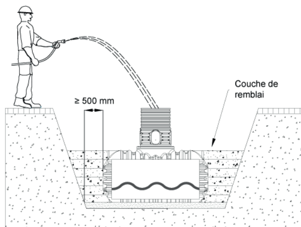
Fig. 33 : Mise en place et remplissage – COMPACT, PROFI
