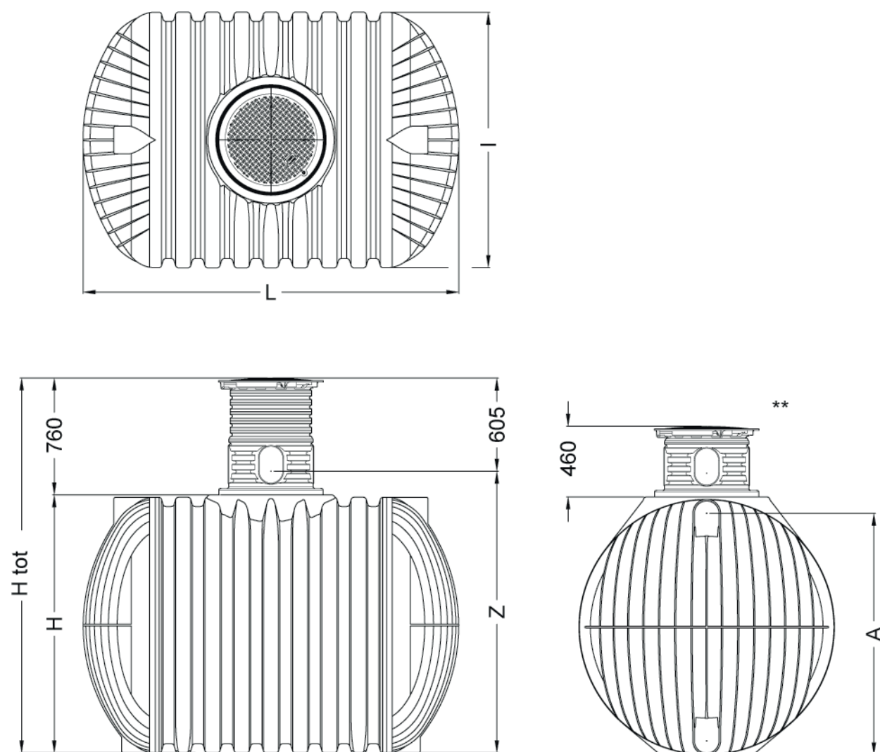
Fig. 10 : Dimensions – PROFI
