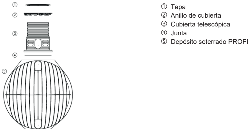
Fig. 20: Componentes – PROFÍ
