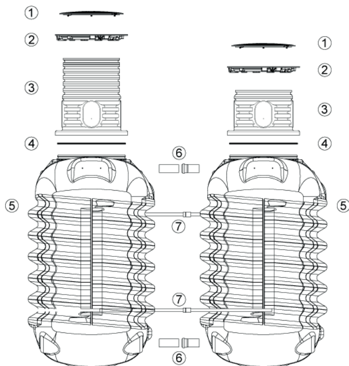
Fig. 18: Componentes – MODULARIS
