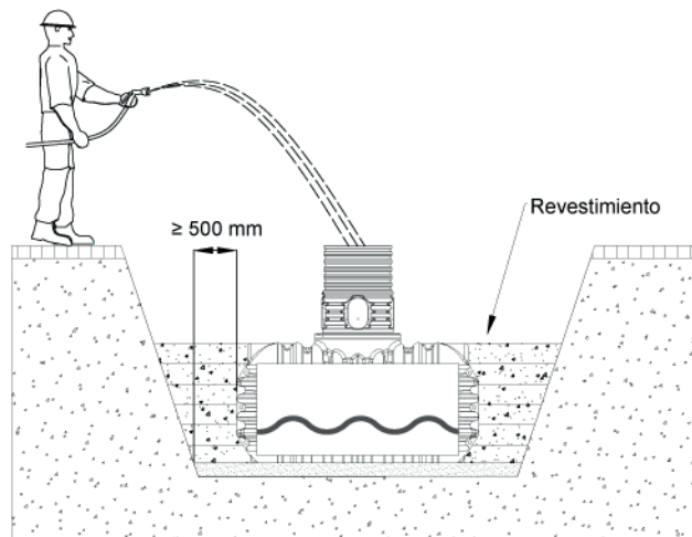
Fig.33: Inserción y relleno – COMPACT, PROFI
