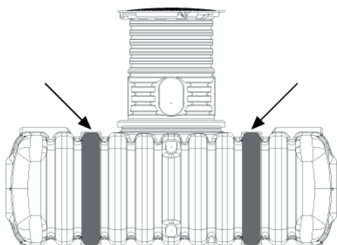
Fig.12: Vista en sección de los tubos de soporte – FLAT S/M
